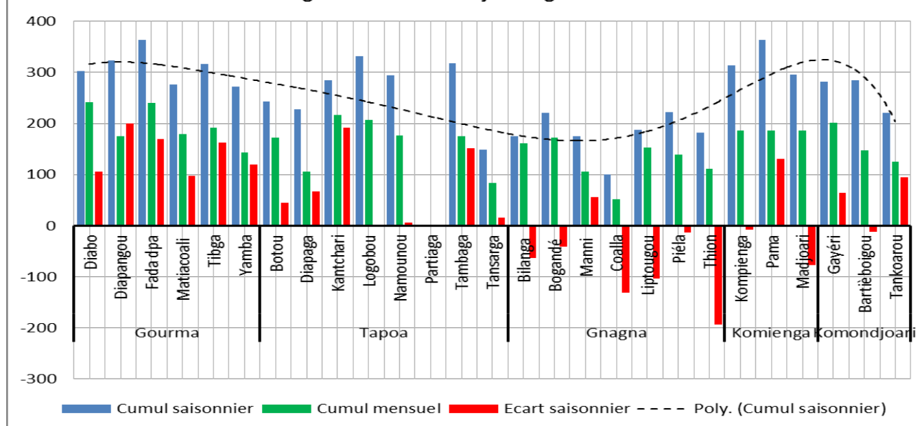
Fig1:Pluviométrie de juin Région de l'Est
